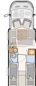
T 7055 EBL 5 soveplasser
