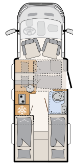
T 6815 EB 5 soveplasser
