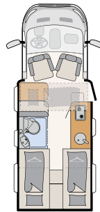
T 6615 EB 4 soveplasser
