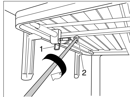
Bilde 150 Høydejustering
