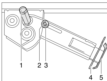
Bilde 39 Støttebein
