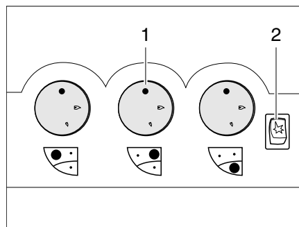
Bilde 323 Brytere for gasskomfyr (med piezo-tenningsknapp)
