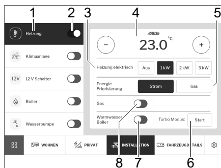
Bilde 274 Varmeanlegg
