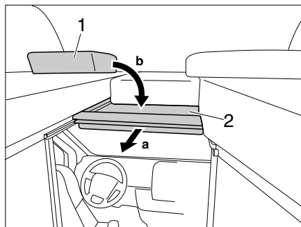
Bilde 60 Førerhuskillevegg
