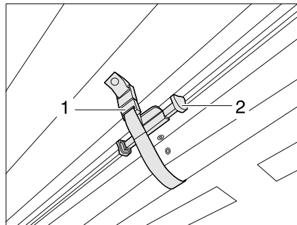
Bilde 14 Sikre blendingsfoldegardinen for frontruten
