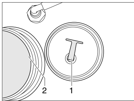
Bilde 350 Blindplugg
