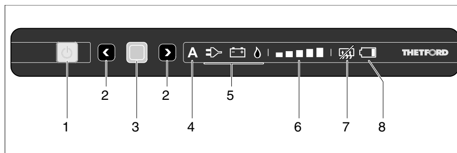
Bilde 337 Betjenings- og visningselementer for kjøleskapet (Thetford uten SES)
