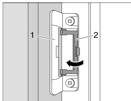
Bilde 345 Låse i luftestilling
