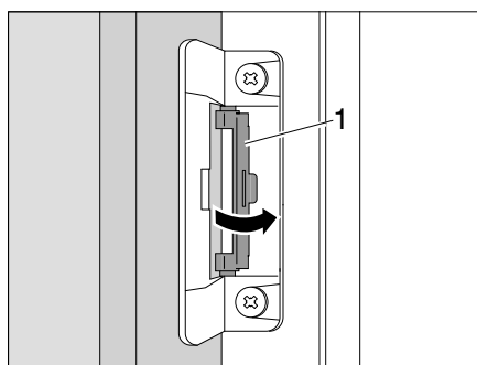
Bilde 346 Dreii låsen tilbake i utgangsstilling
