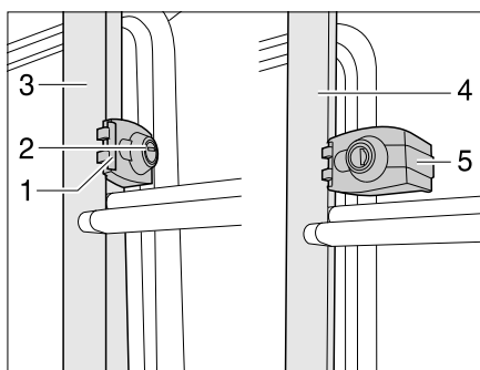
Bilde 1 Lås til stige bak
